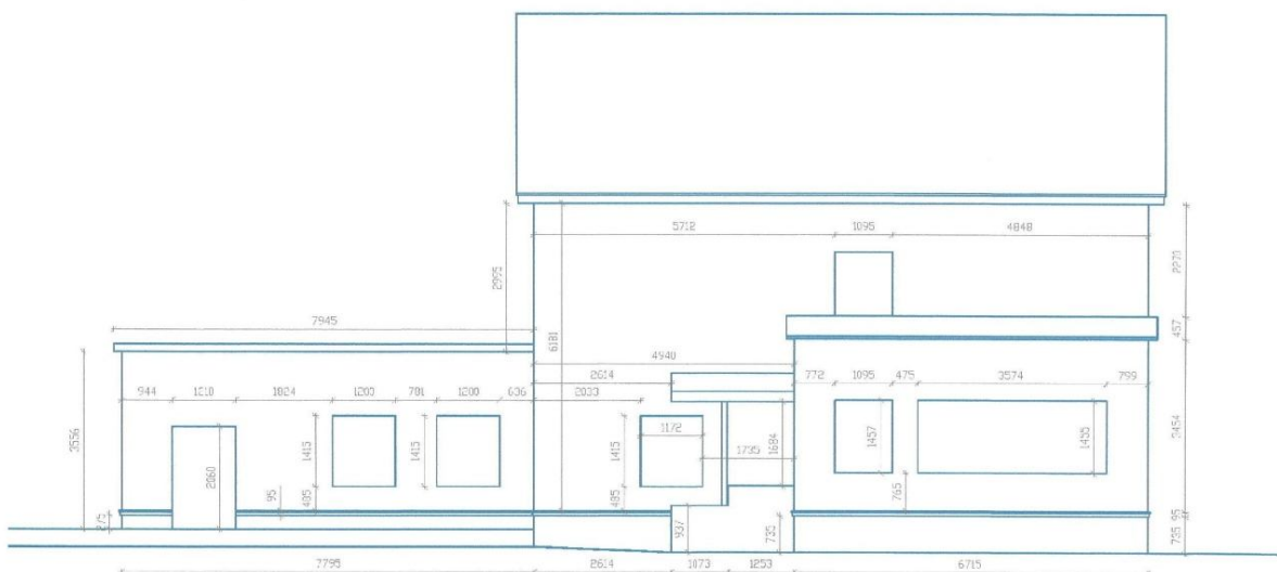
Обмерочный чертёж в осях 1-3
