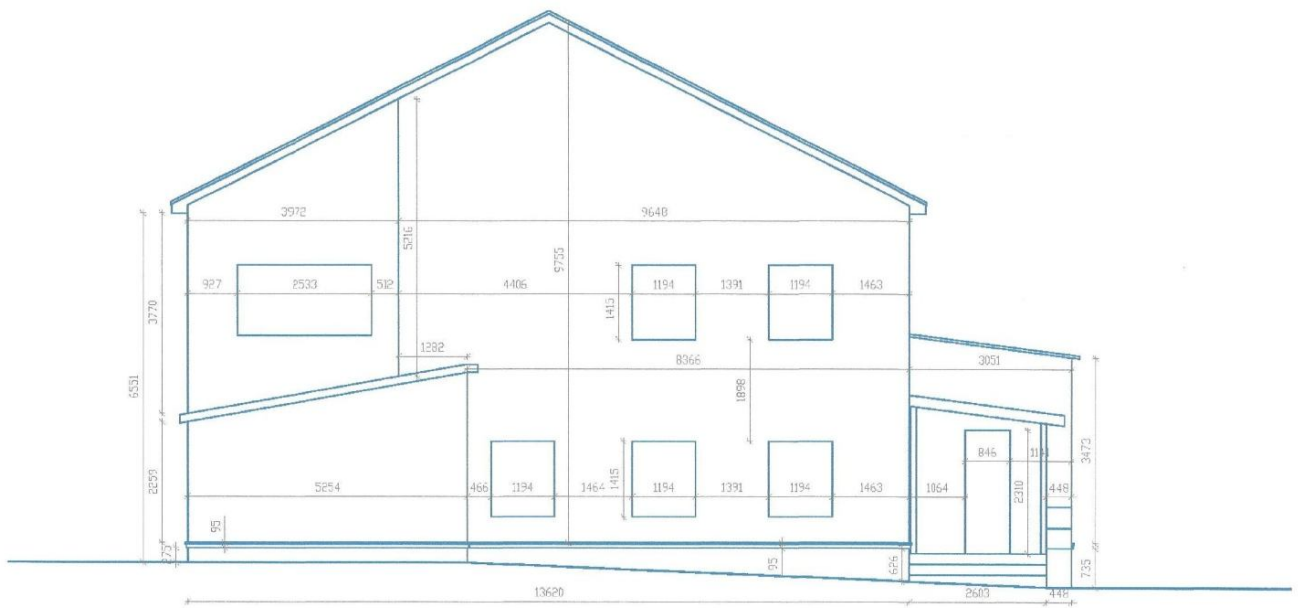
Обмерочный чертёж в осях Г-А
