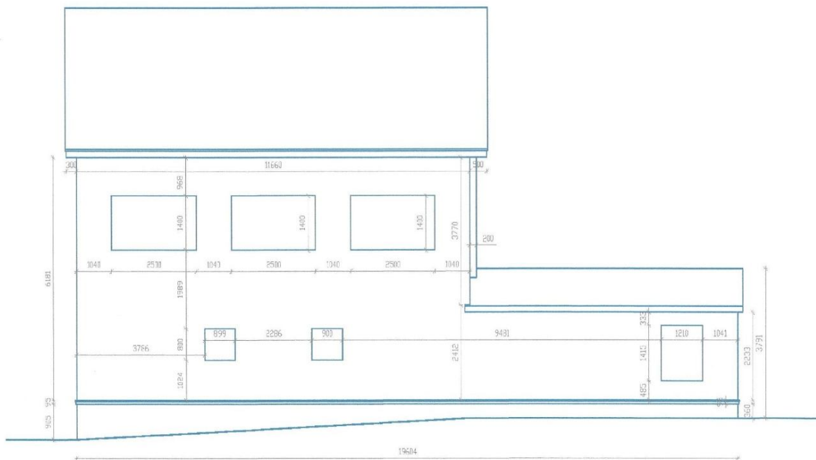
Обмерочный чертёж в осях 3-1
