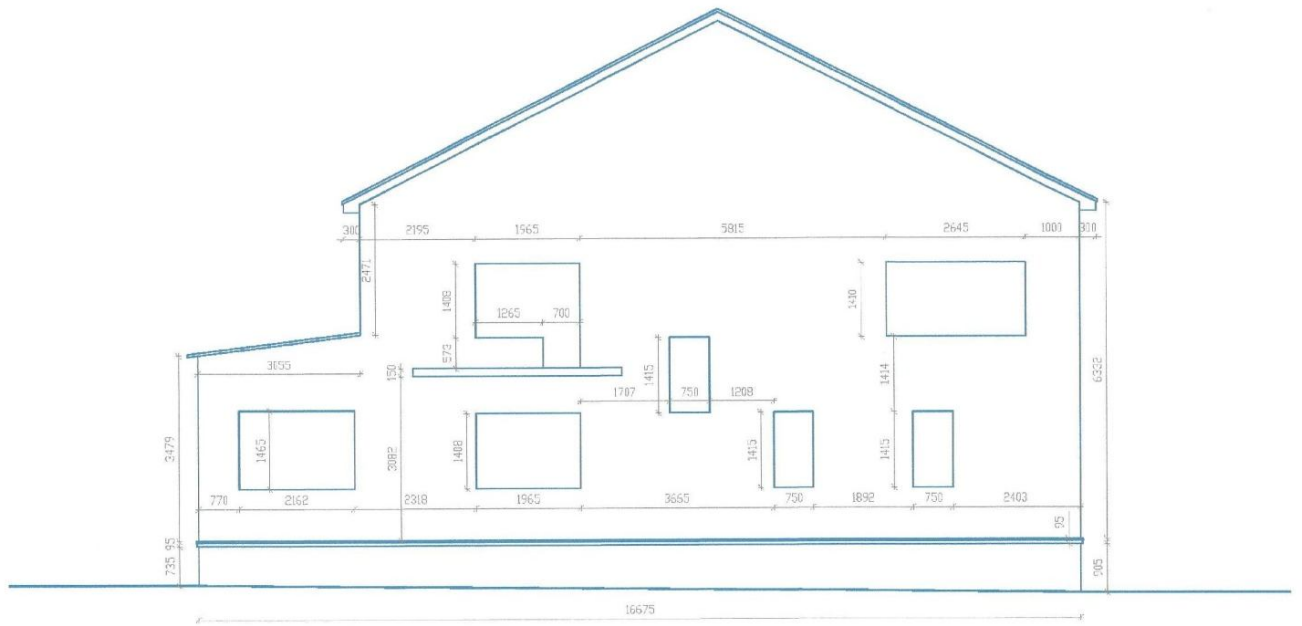
Обмерочный чертёж в осях А-Г
